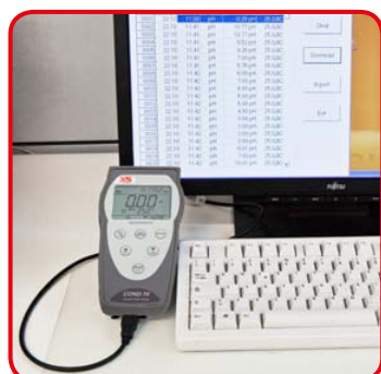
Collegamento a PC con cavo USB
