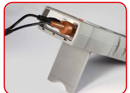
Connettori di collegamento sonde
